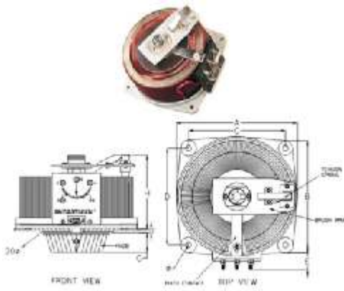
F1 - Variac - Single Phase Flush Back of Panel, Open Input 230V A.C., Output 270V A.C., 50-60Hz
